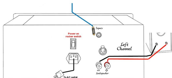
•Conexión a amplificadores monoaurales
