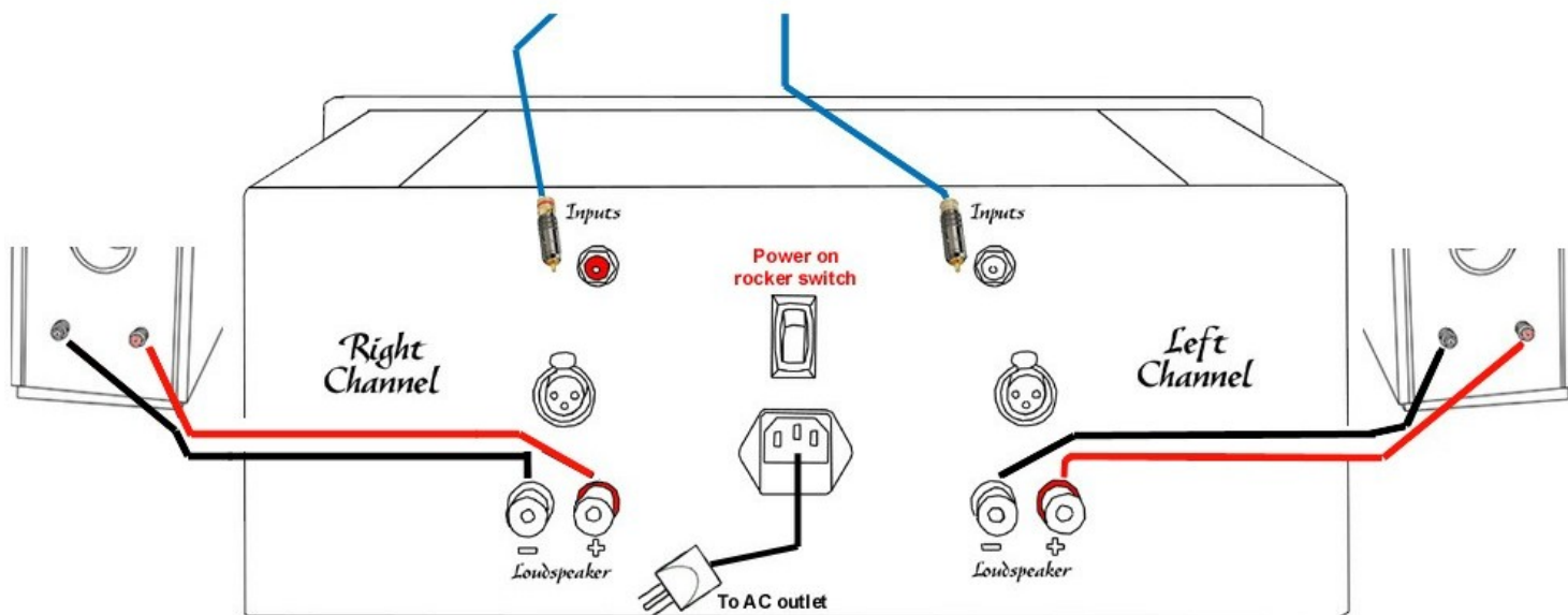
•Conexión a amplificador estéreo
